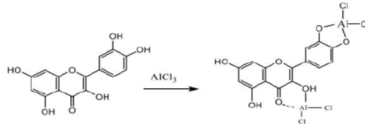
Gambar 2. Reaksi antara flavonoid dengan \text{AlCl}_3 (Suharyanto dan Prima, 2020)
