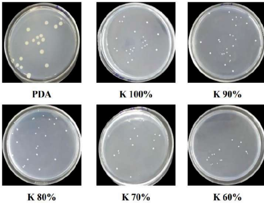
Gambar 1. Hasil pengamatan makroskopis media PDA dan Alternatif media saripati sukun
