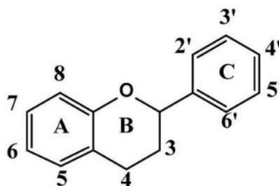
Gambar 6. Struktur umum flavonoid
