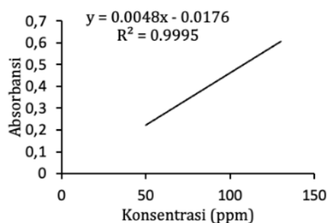
Gambar 5. Kurva hubungan konsentrasi dengan absorbansi kuersetin
