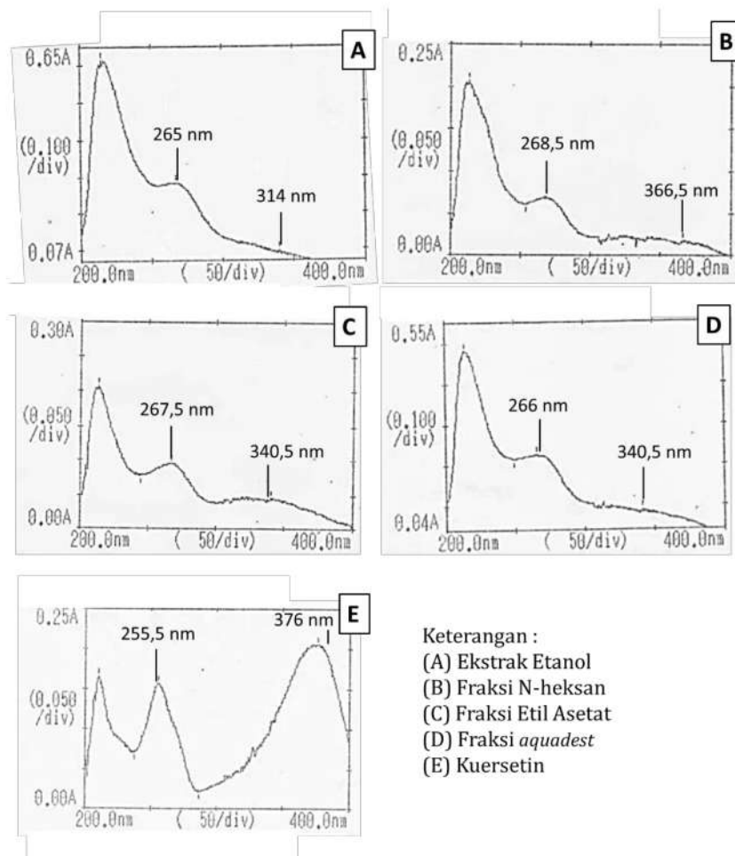
Gambar 4. Spektrum flavonoid dari ekstrak dan fraksi bunga pepaya jantan
