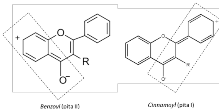
Gambar 3. Struktur benzoyl dan cinnamoyl pada flavonoid
