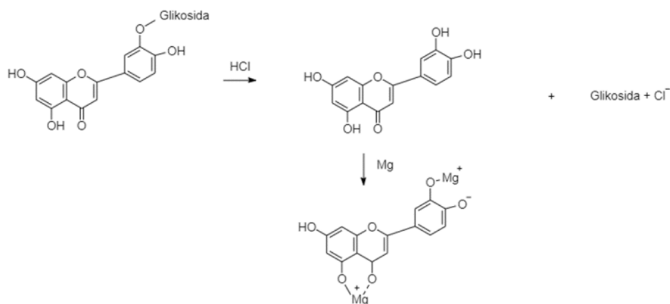
Gambar 1. Uji flavonoid dengan reaksi Wilstater
