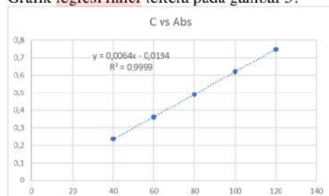
Gambar 3. Kurva Baku Flavonoid (Konsentrasi VS Absorbansi)
