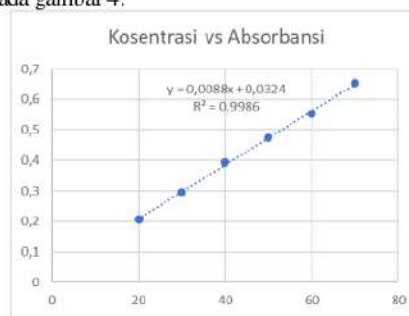
Gambar 4. Kurva Baku Fenol (Konsentrasi VS Absorbansi)
