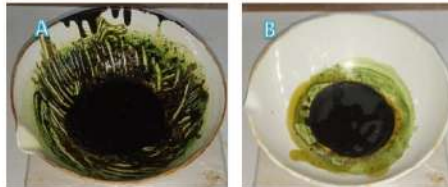
Gambar 2. Ekstrak Herba Suruhan; A: Ekstrak Kasar, B: Ekstrak Terpurifikasi
